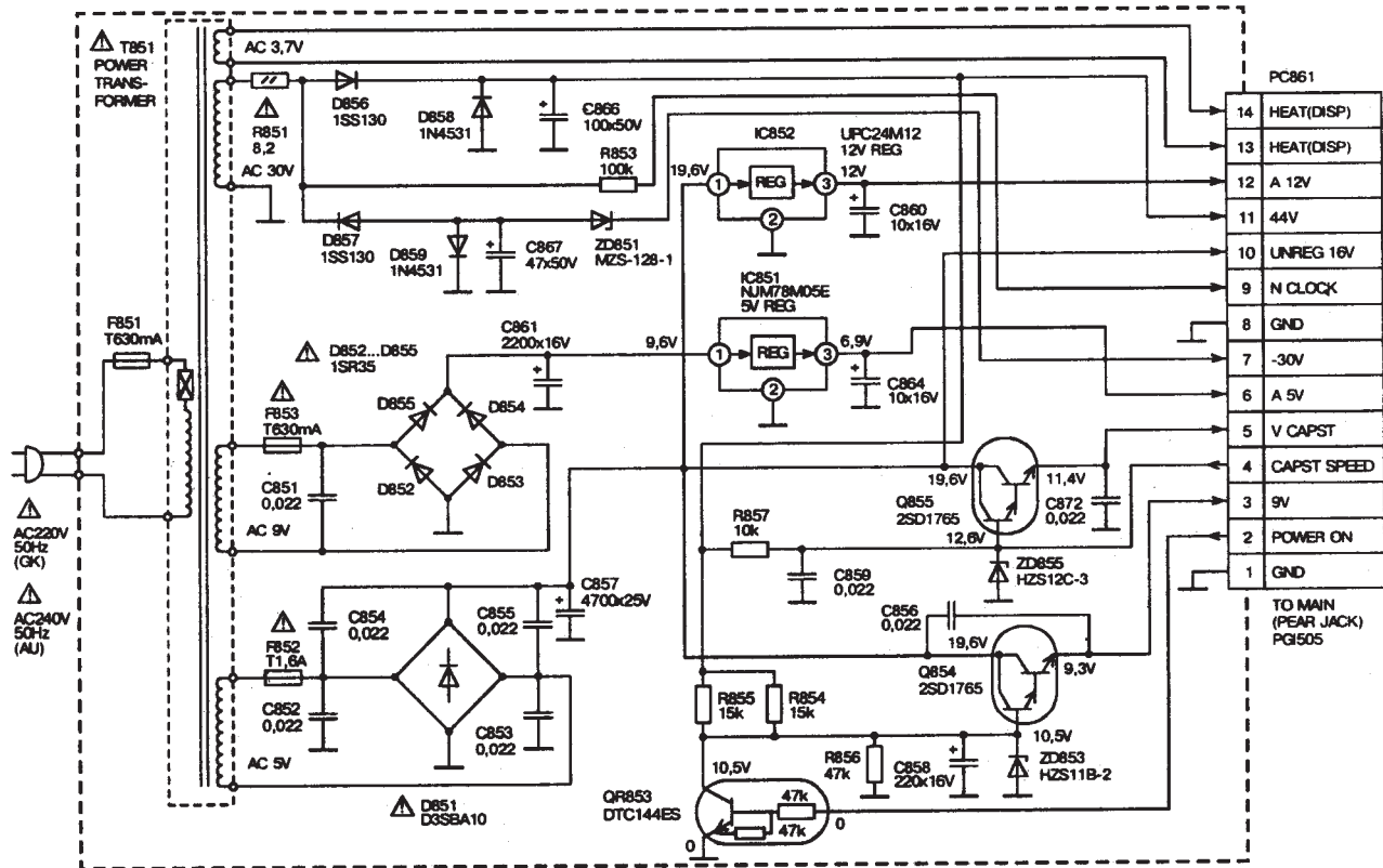
Принципиальная схема источника питания видеомэгнитофонов VT-410/415/416E/M757/M827.
